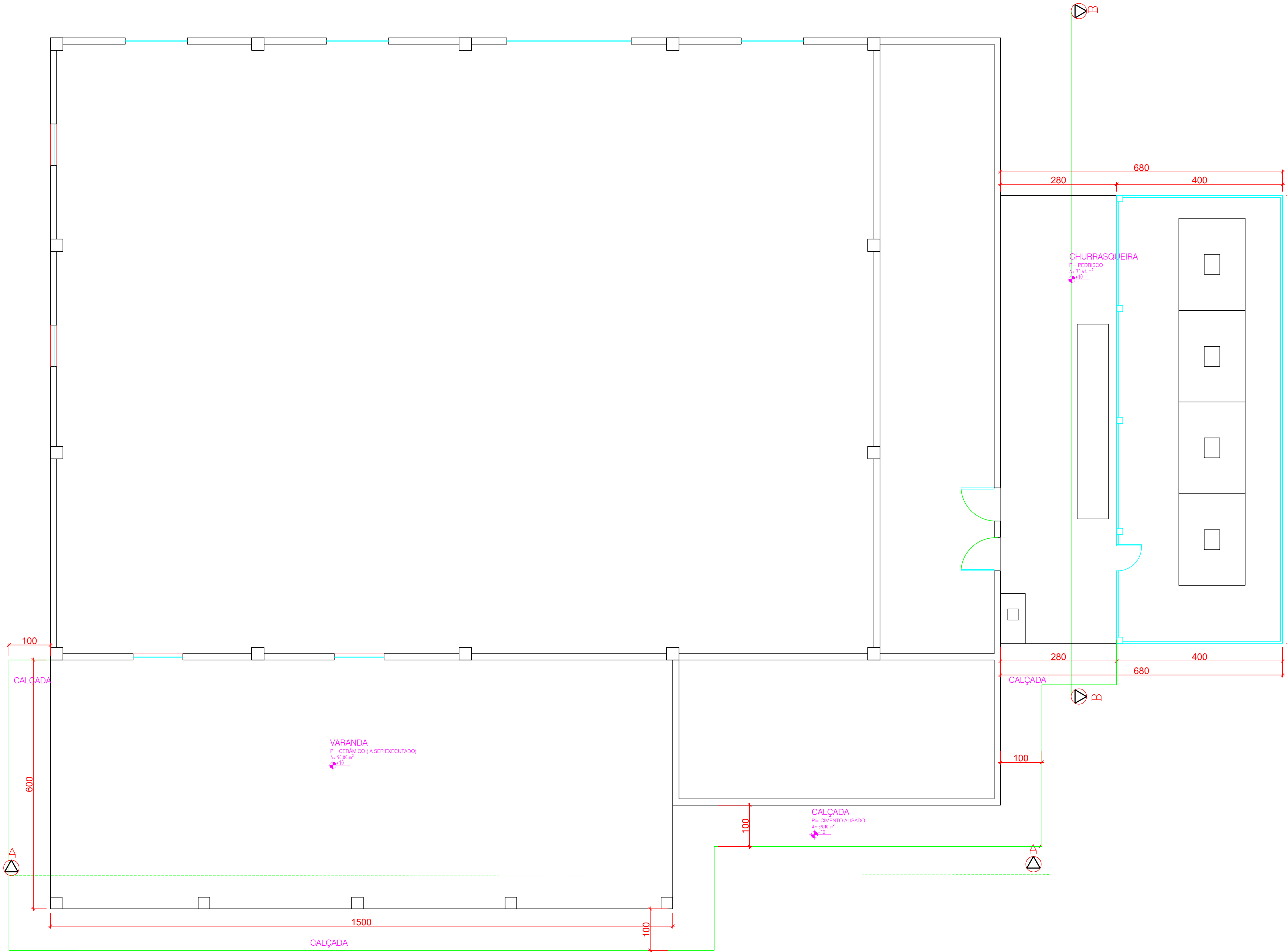
PLANTA-BAIXA ESCALA 1/50
